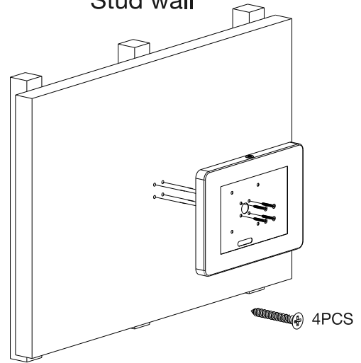
Stud wall
